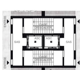
Ascenseurs et escaliers entrée/sortie piétons
